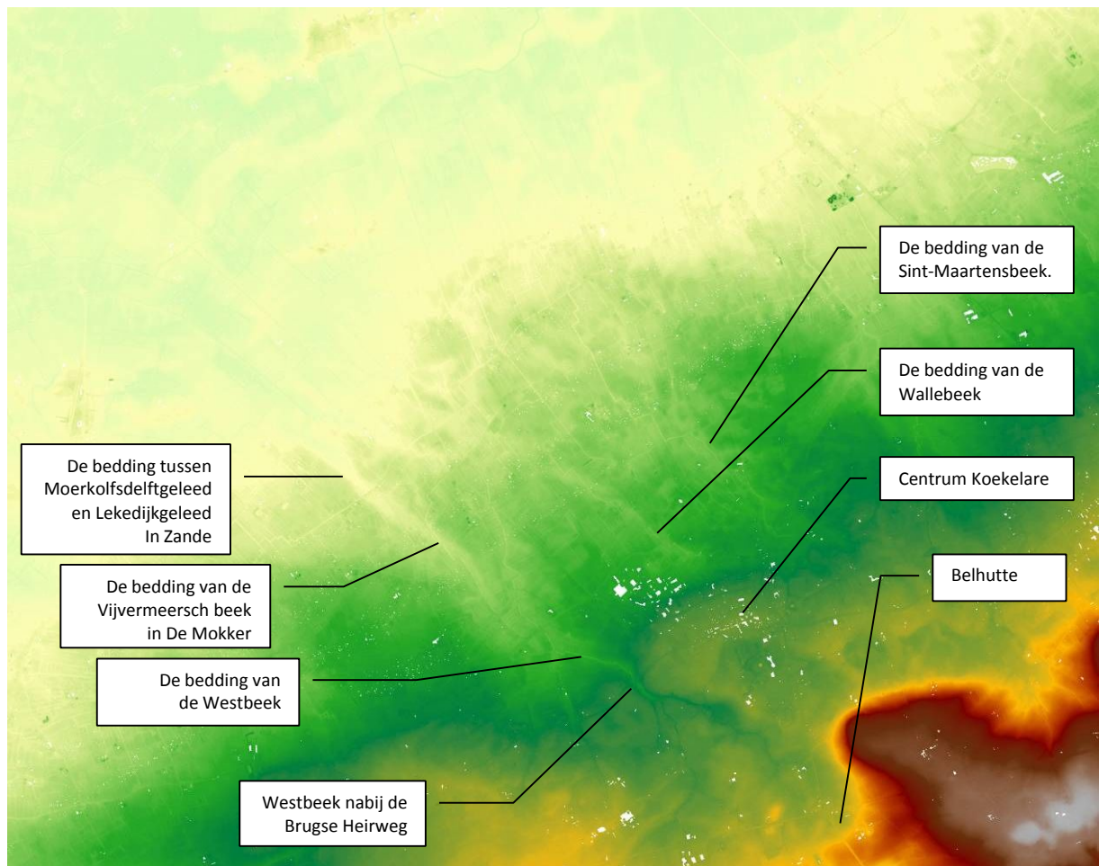
Digitaal hoogtemodel 42 (raster 5m) van het noorden van Koekelare. Bovenaan Gistelmoer, onderaan rechts de Koekelareberg.
