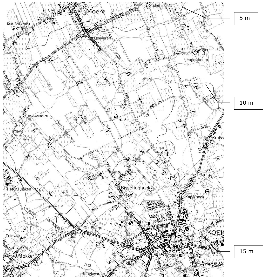
Fragment van de topografische kaart waarbij de hoogtelijnen van 5 m, 10 m en 15 m een behoorlijk evenwijdig verloop hebben.
