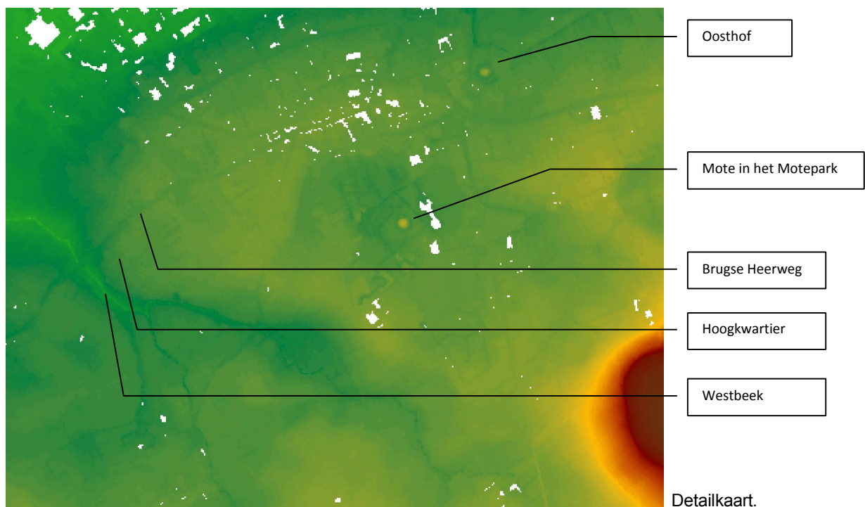
Digitaal hoogtemodel 42 (raster 5m) van het noorden van Koekelare. Bovenaan Gistelmoer, onderaan rechts de Koekelareberg.
