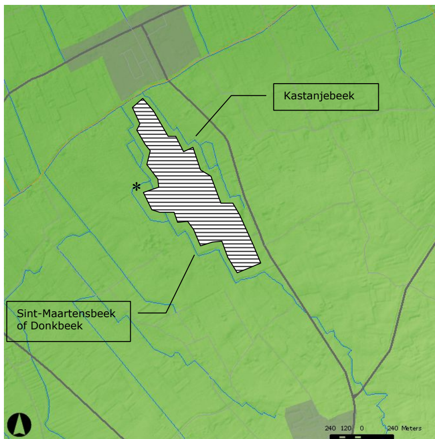
De depressie van de Sint-Maartensbeek tussen het huidige tracé en zijn noordwestelijke evenknie, de Kastanjebeek. Hoogtemodel (raster 100 m) – Relief - GISWest 2009.
